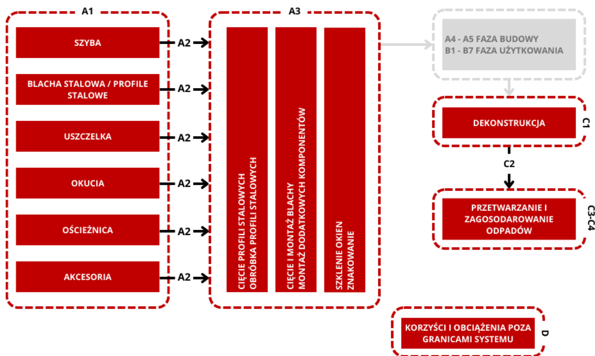
Rysunek 5.1: Granice systemu dla charakterystyki środowiskowej drzwi stalowych płaszczyznych
